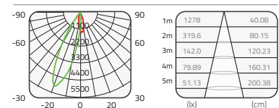
CREE 15W±10% 3000K 22° Ra80
