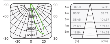
CREE 11W±10% 3000K 20° Ra80
