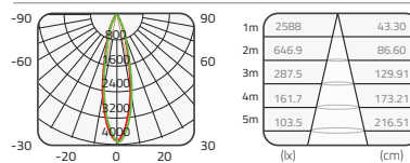
CREE 11W±10% 3000K 24° Ra80
