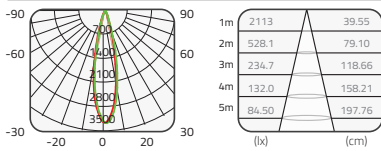
CREE 9W±10% 3000K 22° Ra80
