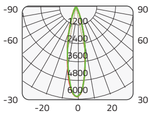
CREE 15W±10% 3000K 24° Ra80
