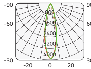
CREE 11W±10% 3000K 24° Ra80
