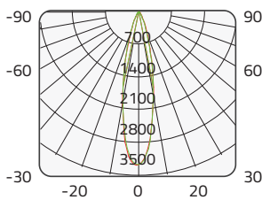
CREE 11W±10% 3000K 24° Ra90
