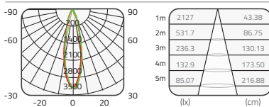
CREE 9W±10% 3000K 24° Ra80
