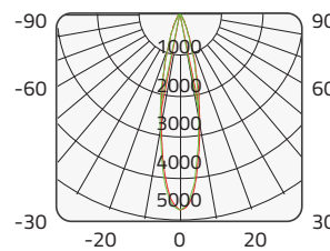
CREE 15W±10% 3000K 24° Ra90
