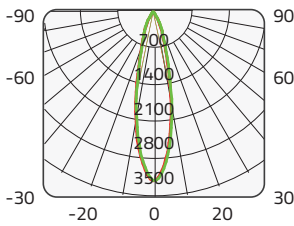
CREE 9W±10% 3000K 24° Ra80
