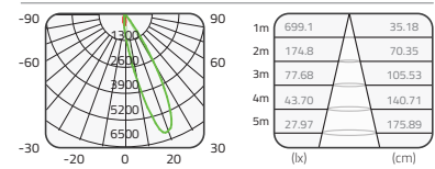
CREE 15W±10% 3000K 20° Ra80
