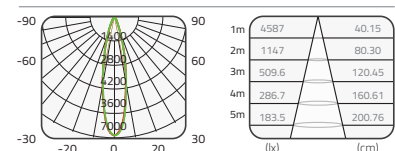
CREE 15W±10% 3000K 24° Ra80
