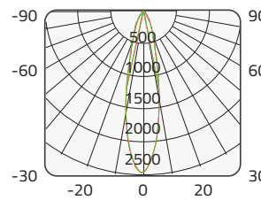
CREE 9W±10% 3000K 24° Ra90
