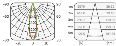
CREE 11W±10% 3000K 22° Ra80
